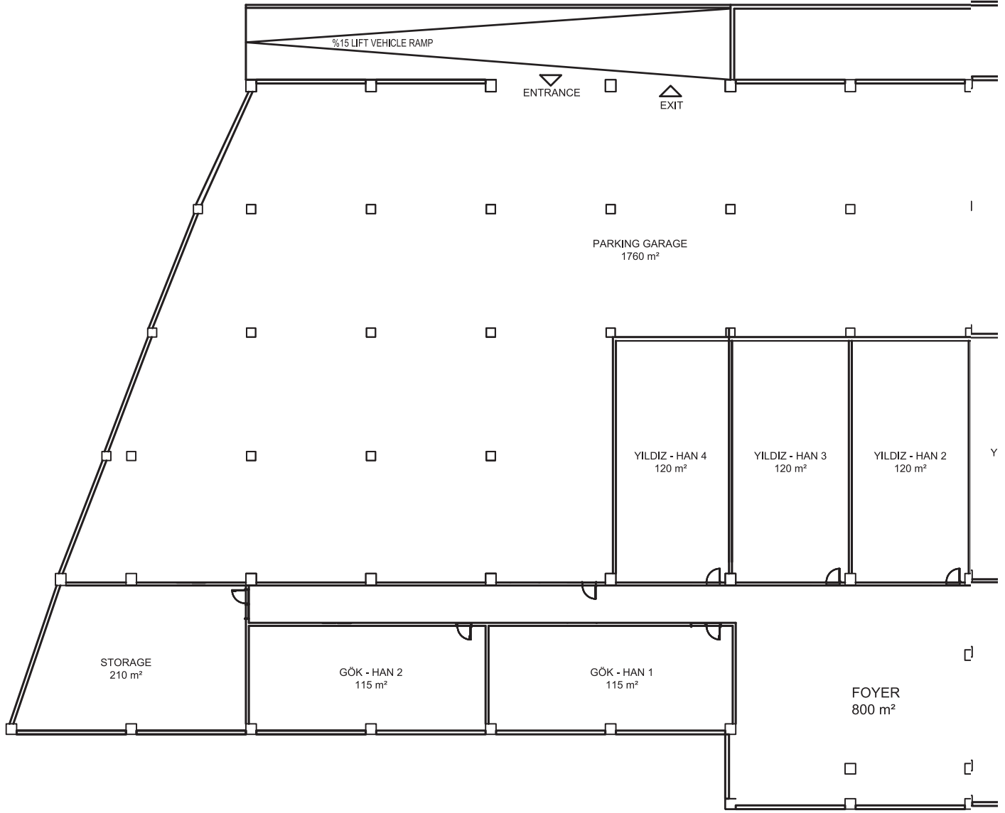
Kongre Merkezi Bodrum Kat Planı Congress Centre Basement Floor Layout
